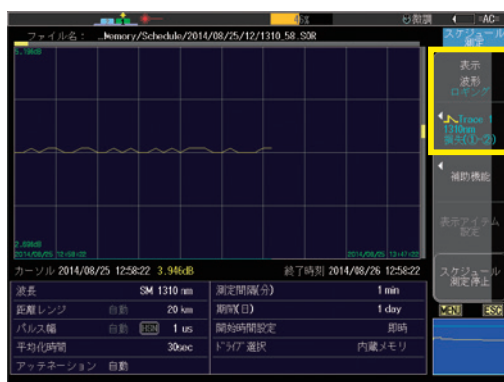
マーカー①・②間の損失値をロギングする例
